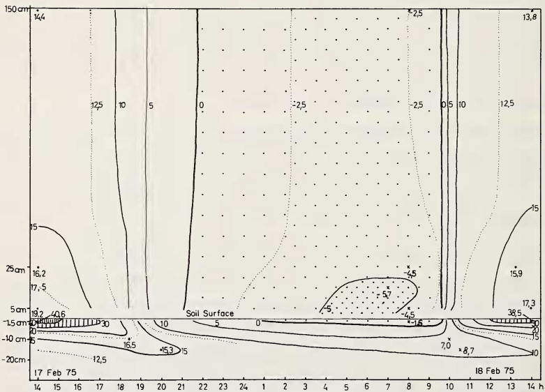
Abb. 4: Tagesgang von Luft- und Bodentemperaturen in den südlichen Cañadas ca. 1 km südöstlich des Parador (2170 m). Oben 16./17. 8. 74 (Sommer), unten 17./18. 2. 75 (Winter).
